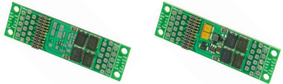
ADAPLU - ohne Niederspannungsquelle ADAPLU15 oder ADAPLU50 - mit Niederspannung 1,5 bzw. 5 V
