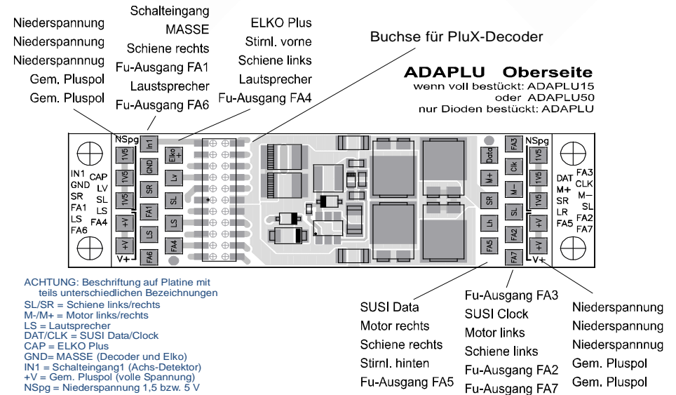
ADAPLU - ohne Niederspannungsquelle ADAPLU15 oder ADAPLU50 - mit Niederspannung 1,5 bzw. 5 V
